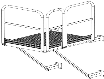
Grundpodest
